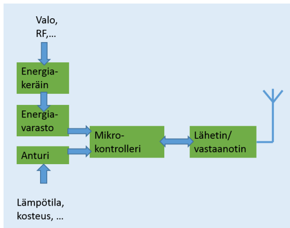
Energiaomavarainen anturi
