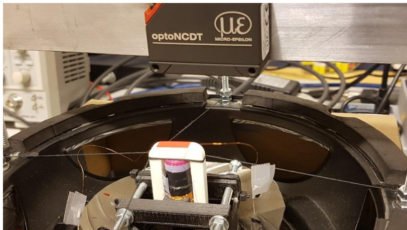
Induktiivisen energiankeräyksen testilaite
